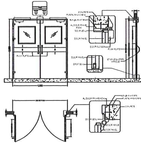
① ประตูบานเปิดคู่ ใช้สำหรับห้องกักกันโดยเฉพาะ
